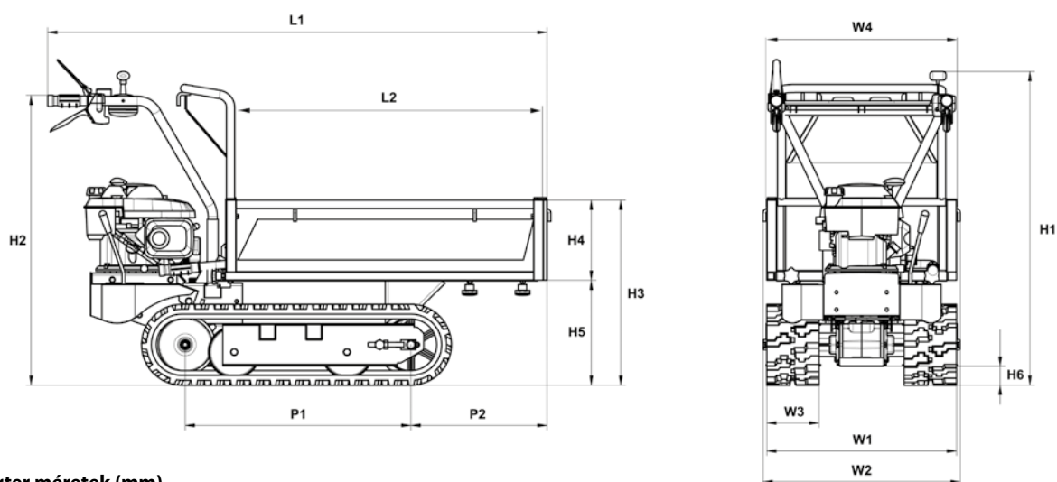
Transzporter méretek (mm)
